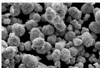
NMC (LiNiCoMnO2)
