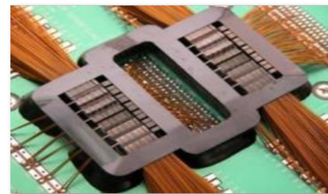
Memory用のプローブカード
