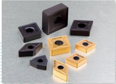
ターニングインサート
