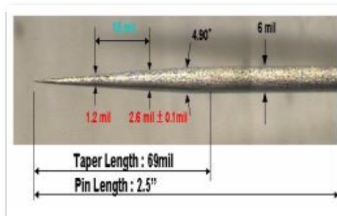
プローブピン
