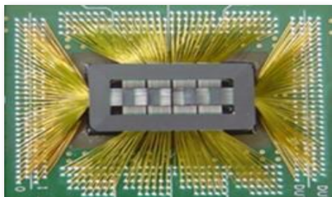
ASIC用のプローブカード
